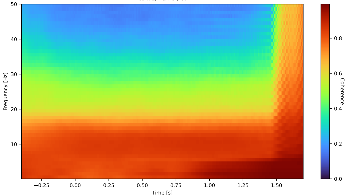
8B (F1) - dPFC (F3)
